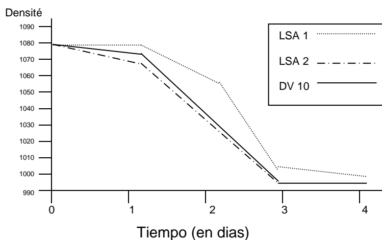
Figura nº1 : pruebas de fermentación alcohólica. Tinas de 12 hl (prueba del CIVC)
