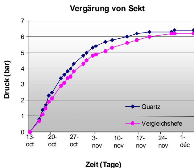
Abbildung 1: Gärversuch bei einem Sektgrundwein aus der Champagne von 2006. Vergleich der Leistungsfähigkeit einer Standardhefe aus der Champagne mit der von QUARTZ . Kinetik des Druckaufbaus.
