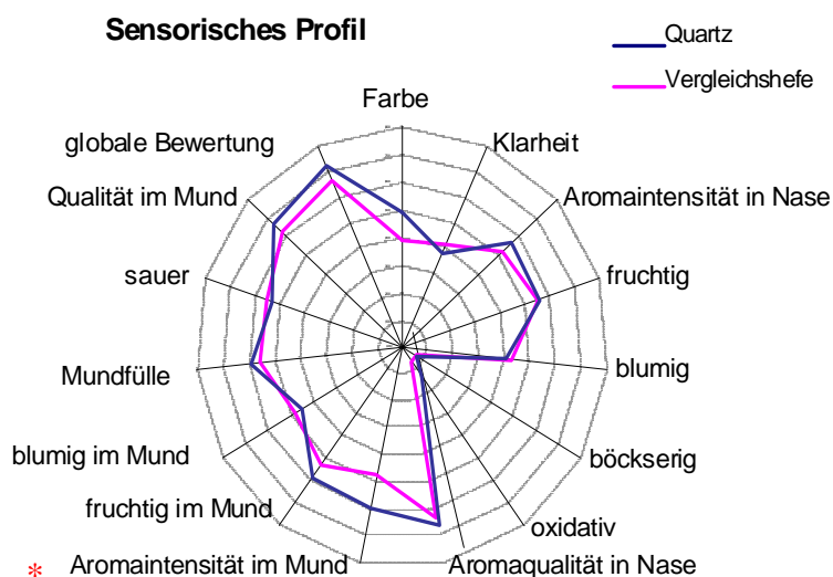
Abbildung 2: Gärversuch bei der Herstellung eines Sektgrundweins aus der Champagne von 2006. Vergleich der Leistungsfähigkeit einer Standardhefe aus der Champagne mit der von QUARTZ . Ergebnisse der sensorischen Analyse.
